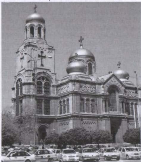
Katedrála Varna
